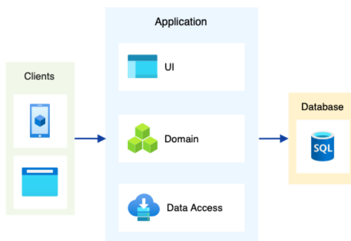
Obrázek 2.1 Monolitická architektura
