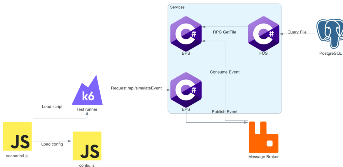
Obrázek 5.4 Diagram scénáře 4
