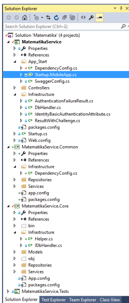
Obr. 11. Struktura backend aplikace.
