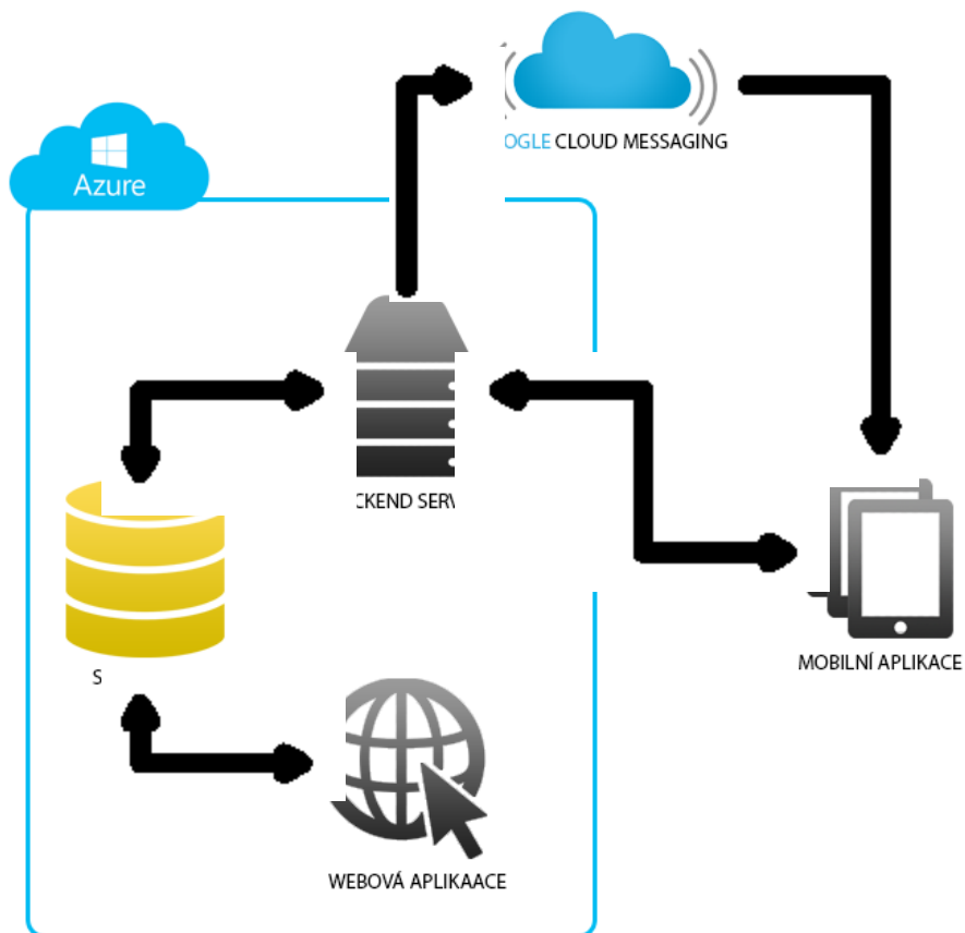
Obr. 9. Schéma jednotlivých aplikací a propojení.
