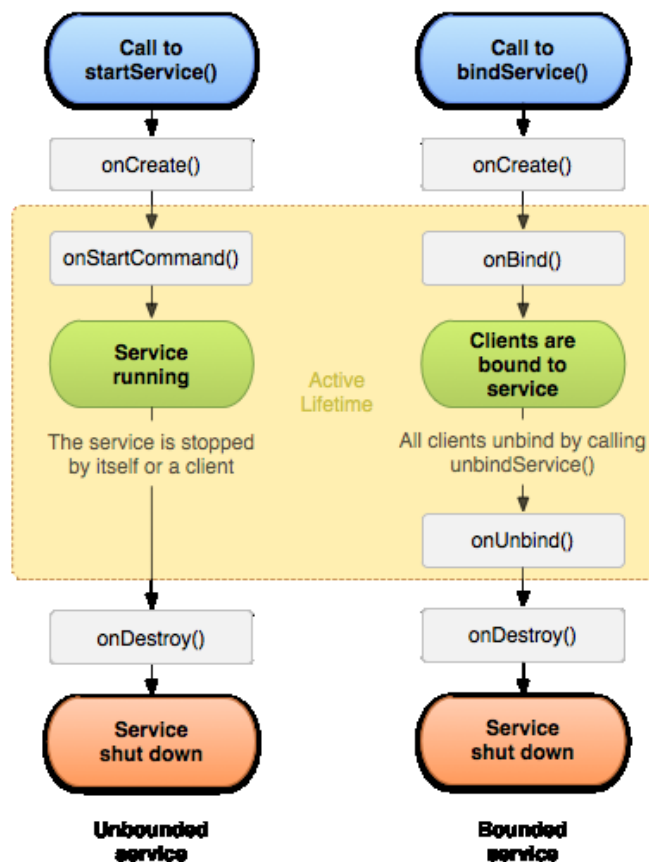
Obr. 2. Životní cyklus služby [8]
