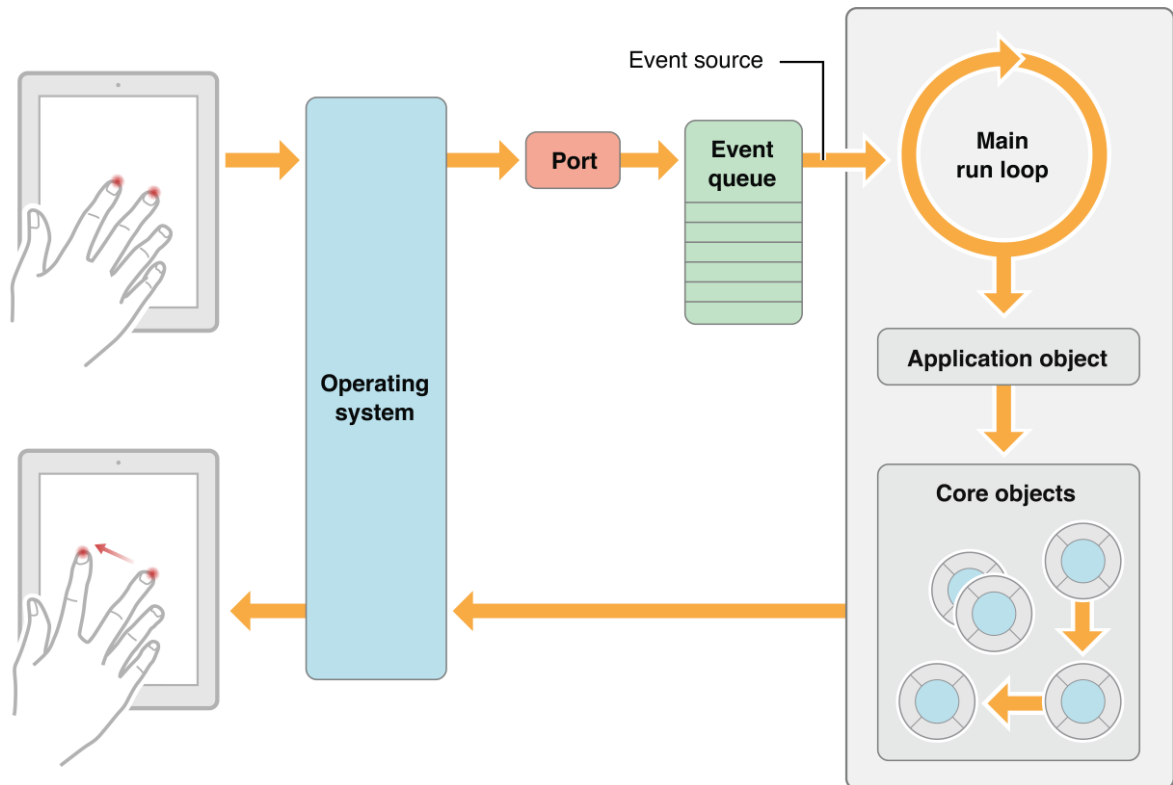
Obr. 6. Ukázka zpracování události v hlavní aplikační smyčce. [15]
