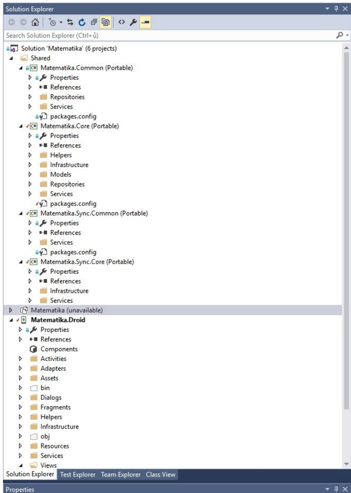
Obr. 12. Struktura projektu mobilní aplikace.
