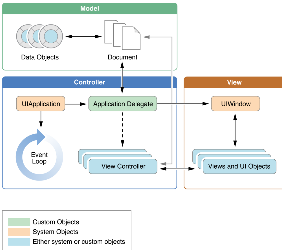
Obr. 5. Struktura iOS aplikace. [15]
