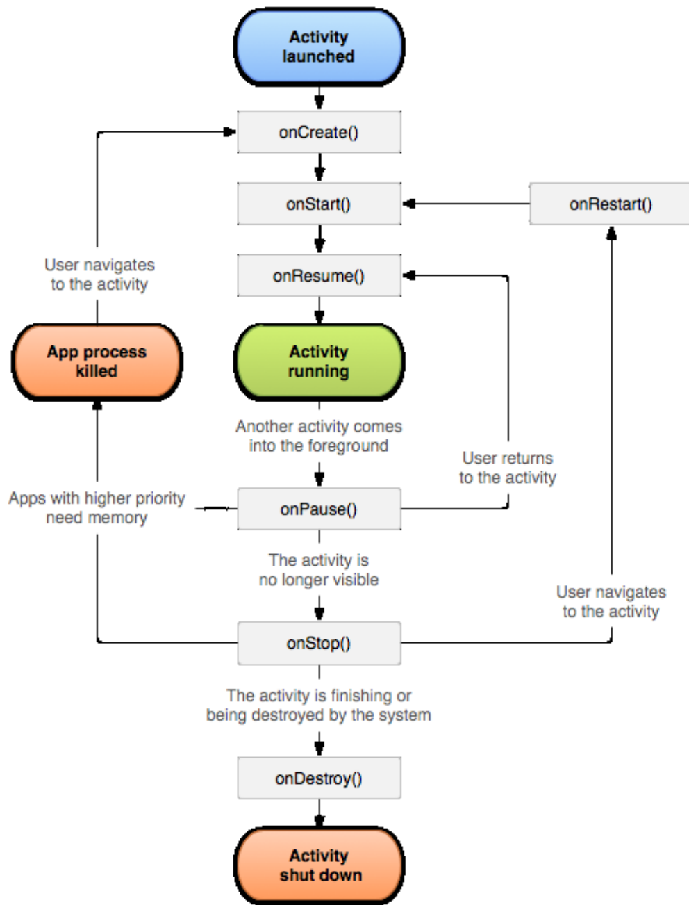
Obr. 1. Životní cyklus aktivity [7]
