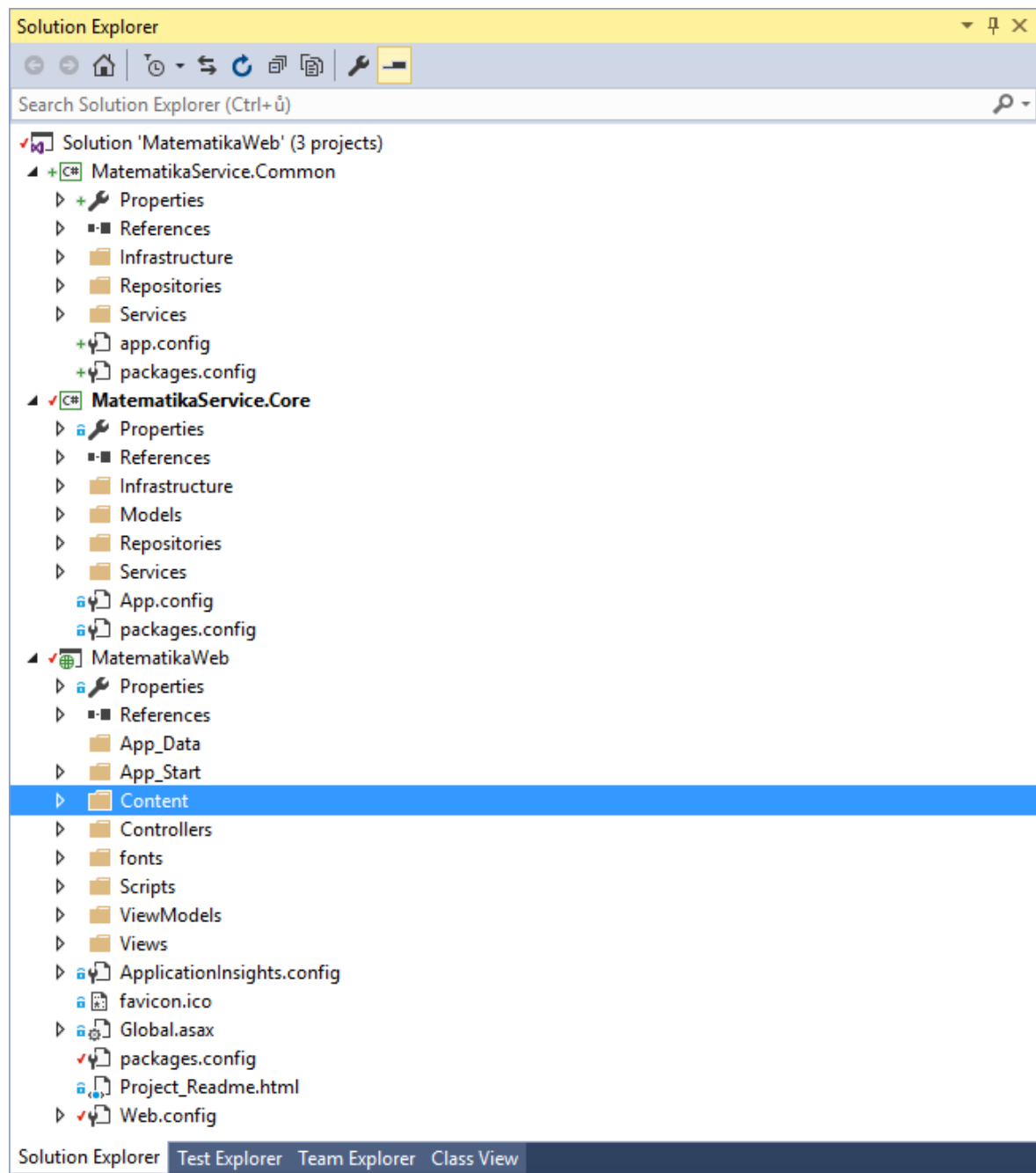
Obr. 13. Struktura webové aplikace.
