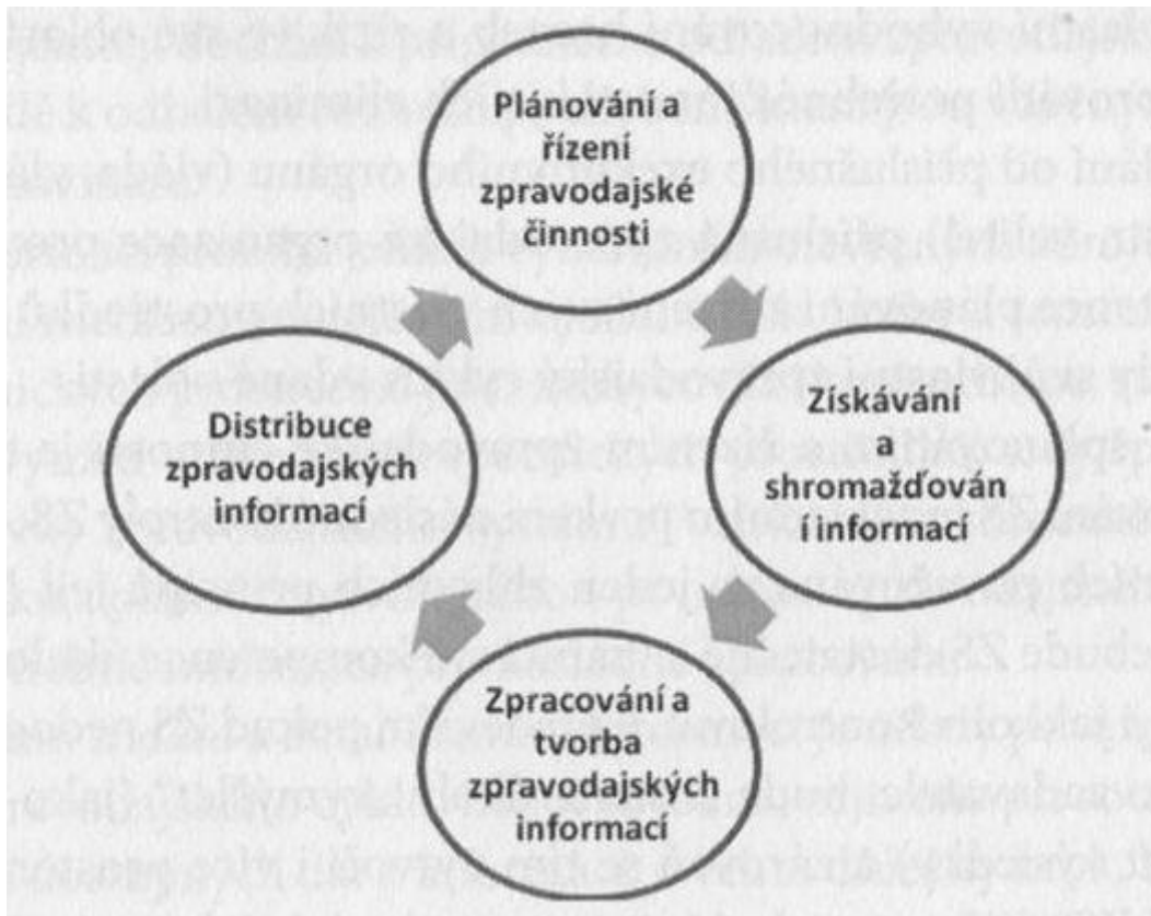
Obr. 5. Zpravodajský cyklus[18]
