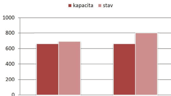
Graf 2 Kapacita a skutečný počet odsouzených
