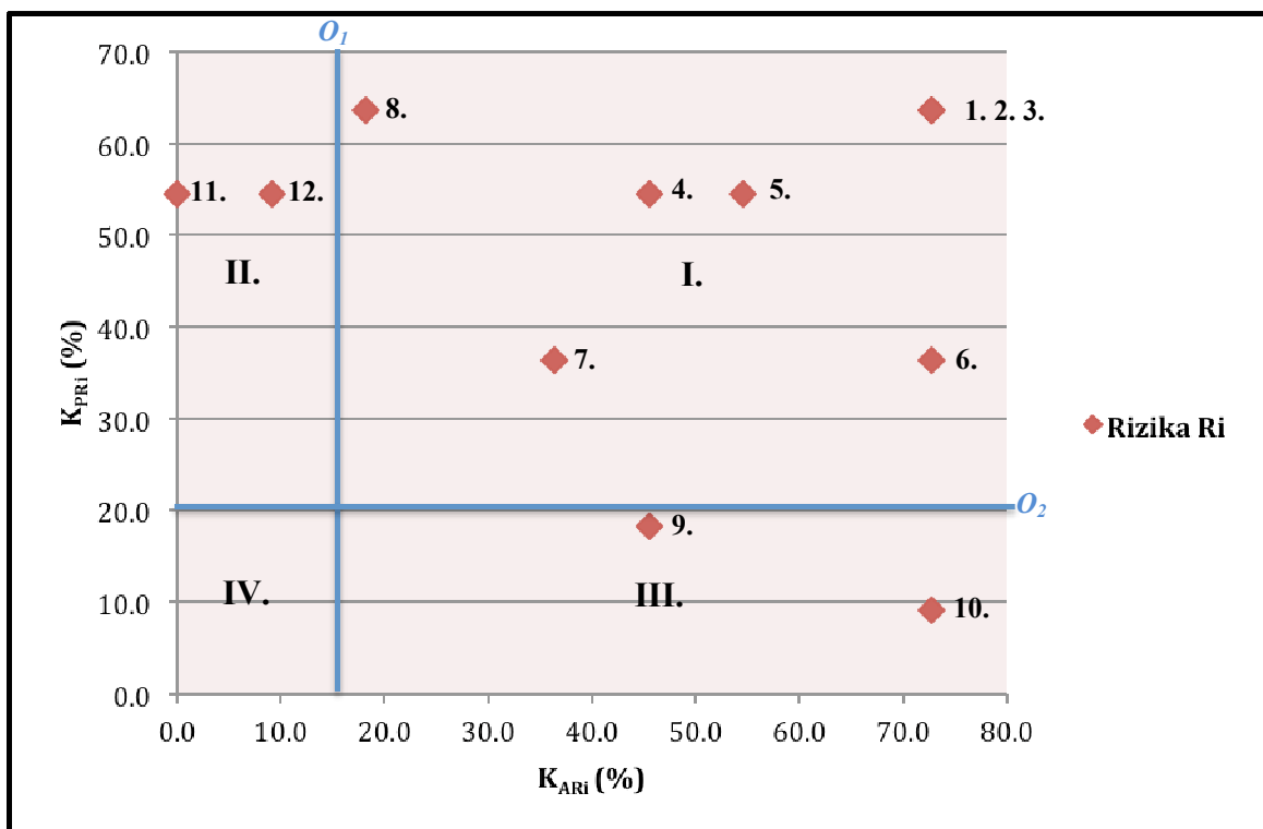
Obr. 25. Výsledný graf analýzy rizik metodou KARS
