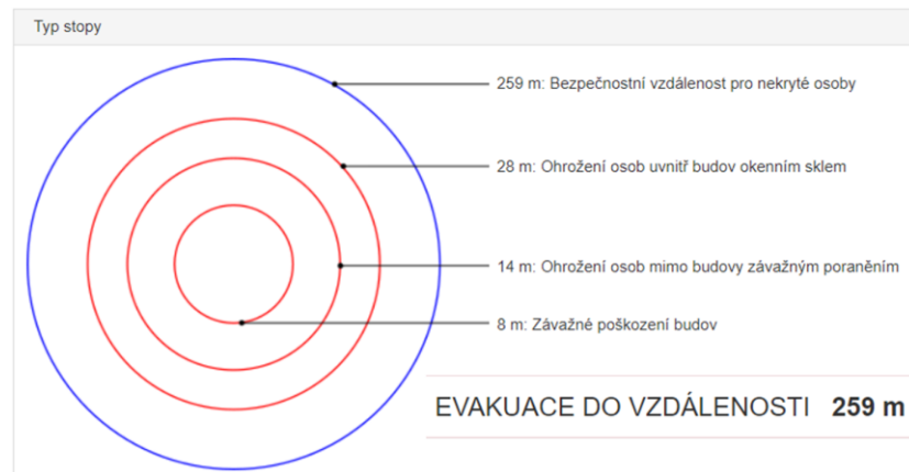
Obrázek 20 – Doporučená vzdálenost. (vlastní zpracování v SW nástroji TerEx, 2024)
