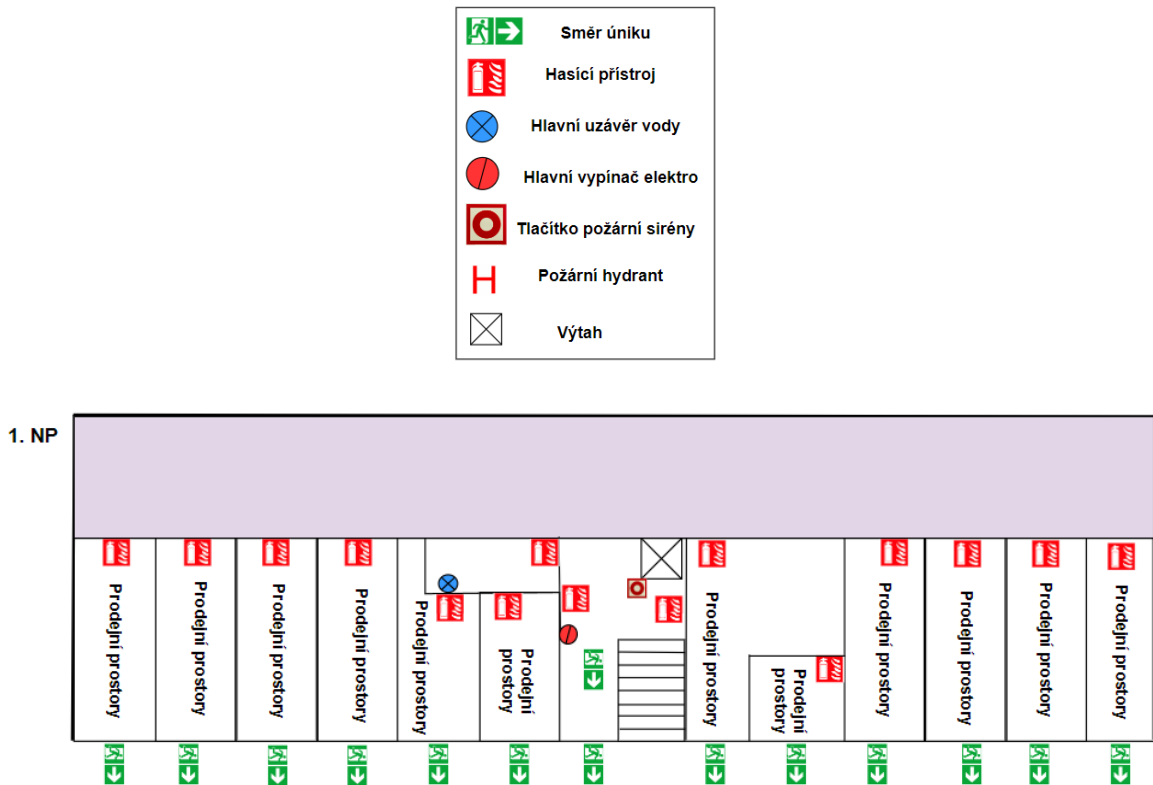
Obrázek 8 – Evakuační plán prvního patra. (vlastní zpracování v Draw.io, 2024)
