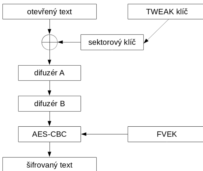
Obr. 2.2 Schéma šifrování sektoru pomocí AES-CBS s Elephant difuzérem[3, 11]
