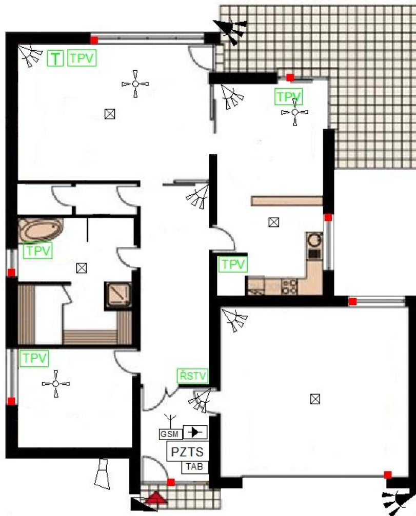
Obrázek 10 – Rodinný dům – půdorys [33]
