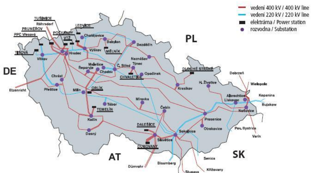
Obrázek 5: Schéma přenosové soustavy (20)
